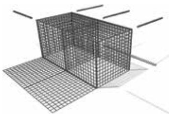
3 Sluiten basis met spiralen
