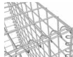
4 Ombuigen uiteinde spiralen
